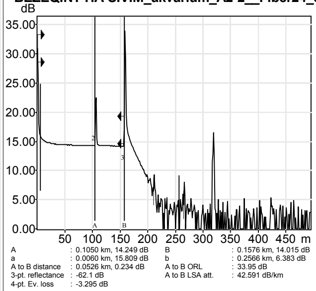
BEZEQINT HA-SIVIM_akvarium_A2-2_Fiber24_8...
