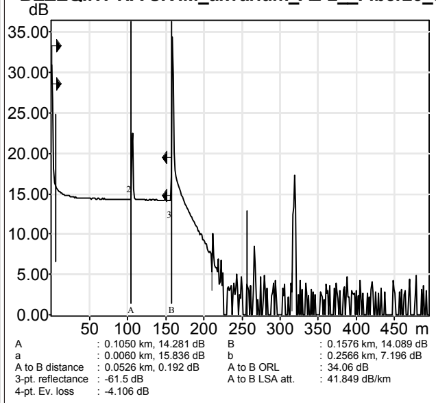
BEZEQINT HA-SIVIM_akvarium_A2-2_Fiber23_8...
